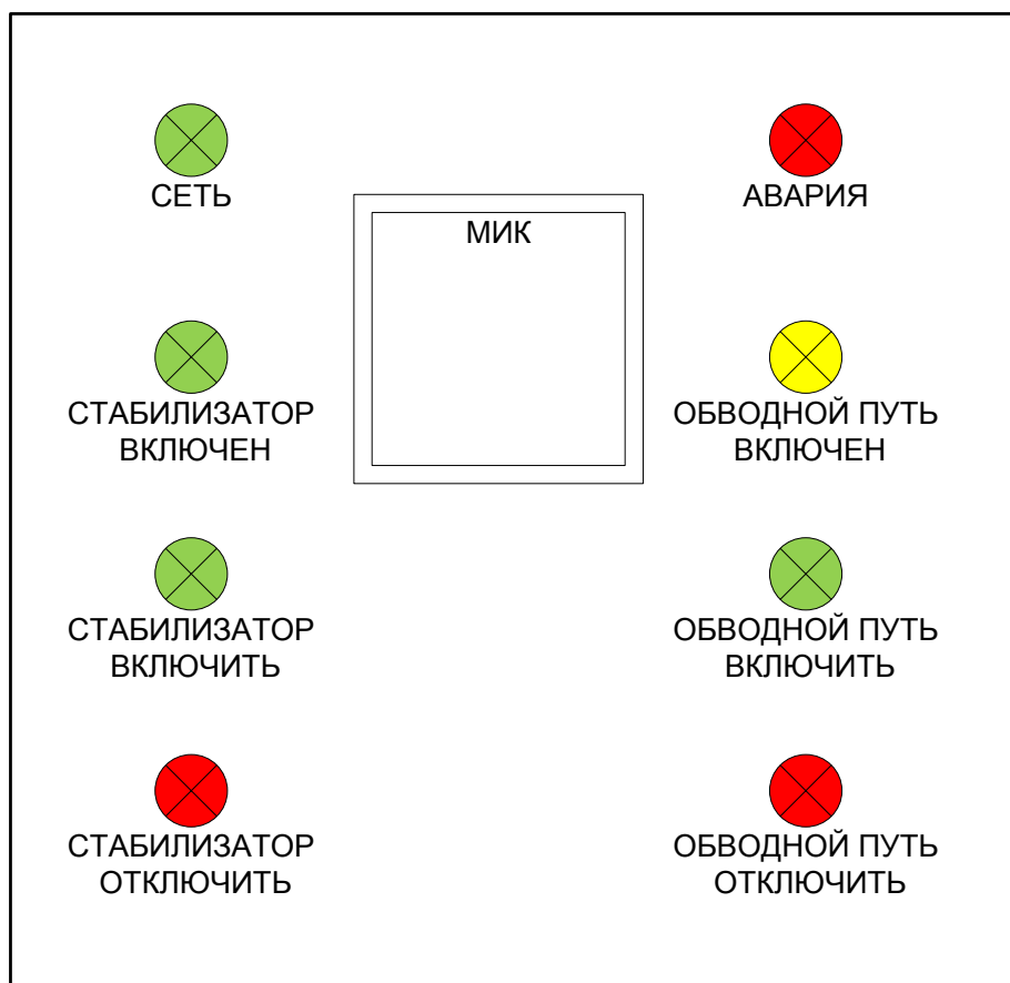
Рисунок 3. Расположение органов индикации и контроля.
